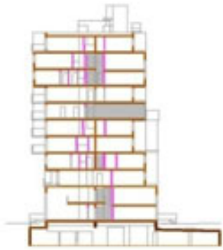
Querschnitt cross sections
