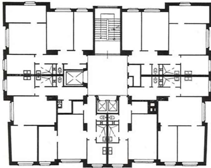
Grundriß eines Normalgeschosses (links) und des Dachgeschosses
