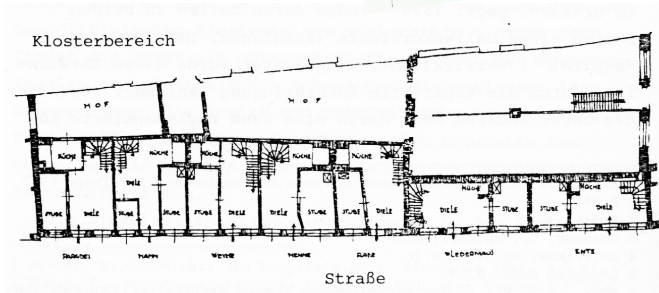
lübeck, armenbuden beim kloster st. anna, grundriss (kloster erbaut 1502-1515), straßenansicht der armenbuden
