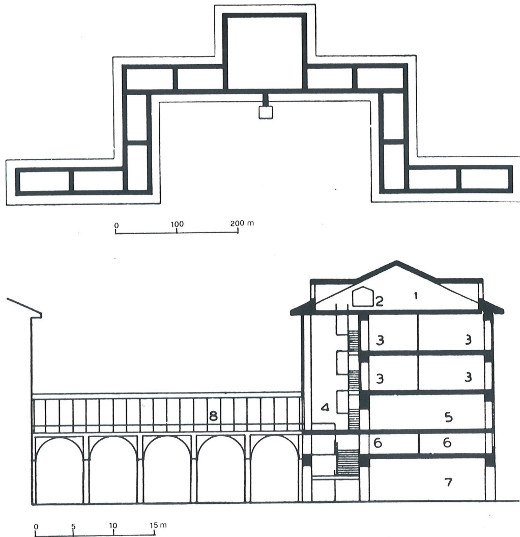
schematischer grundriss einer phalanstère, 1841 ; schematischer querschnitt durch phalanstère
