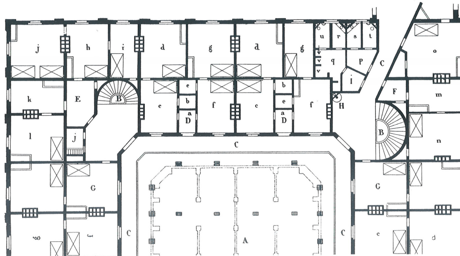
querschnitt und grundriss des hauptgebäudes des familistère in guise
