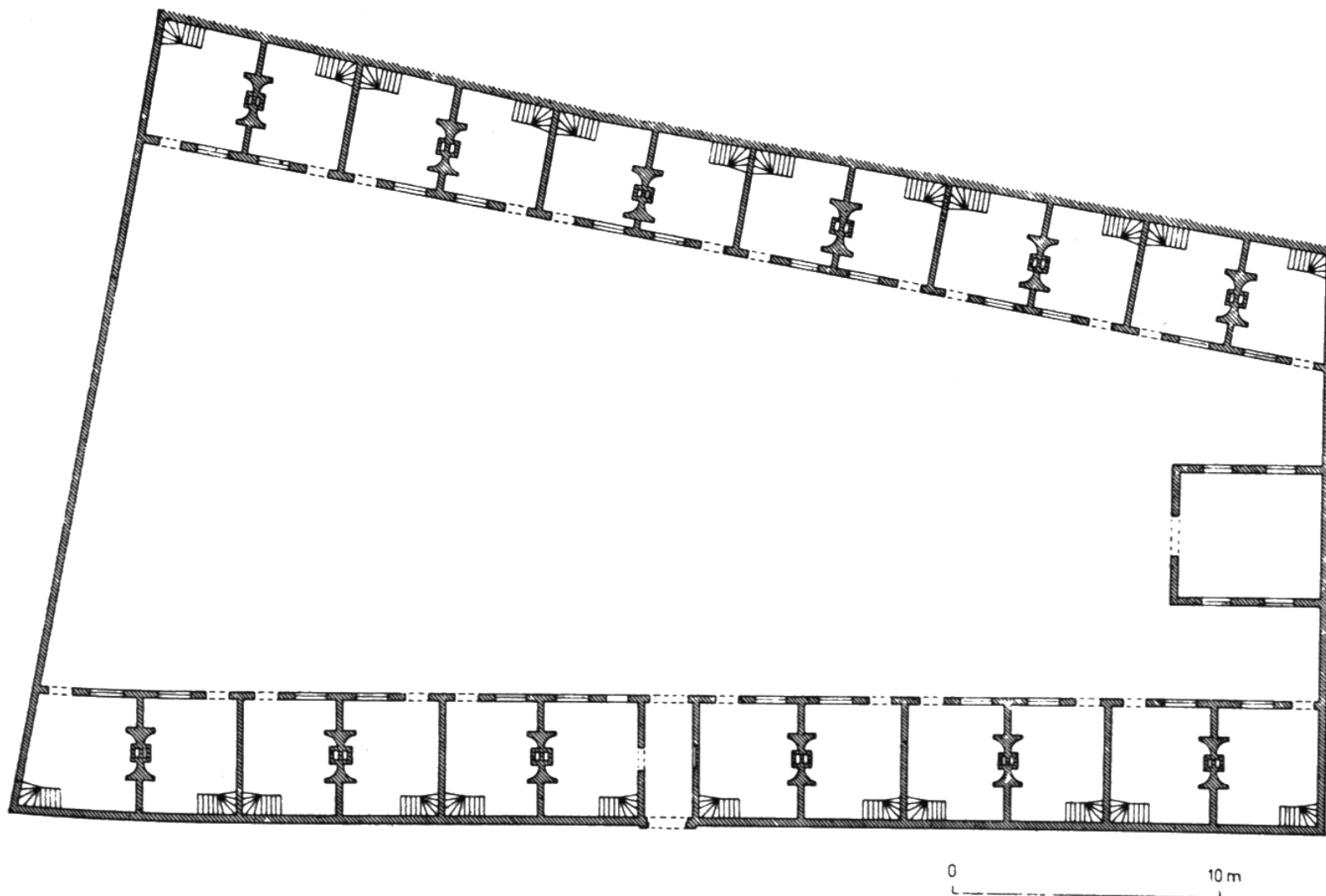
brügge, godshuis meulenaere am nieuwe gentweg, gestiftet 1613, grundriss
