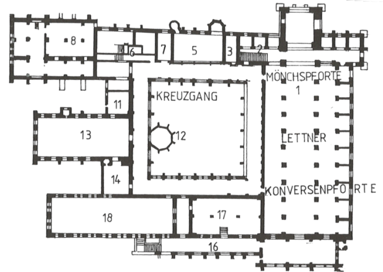
Abb. 3b Maulbronn (gegr. 1147), Grundriß der Klausur (13. Jahrhundert ff.)
