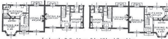
Letchworth: Reihenhäuser, Schaubild und Grundrisse
