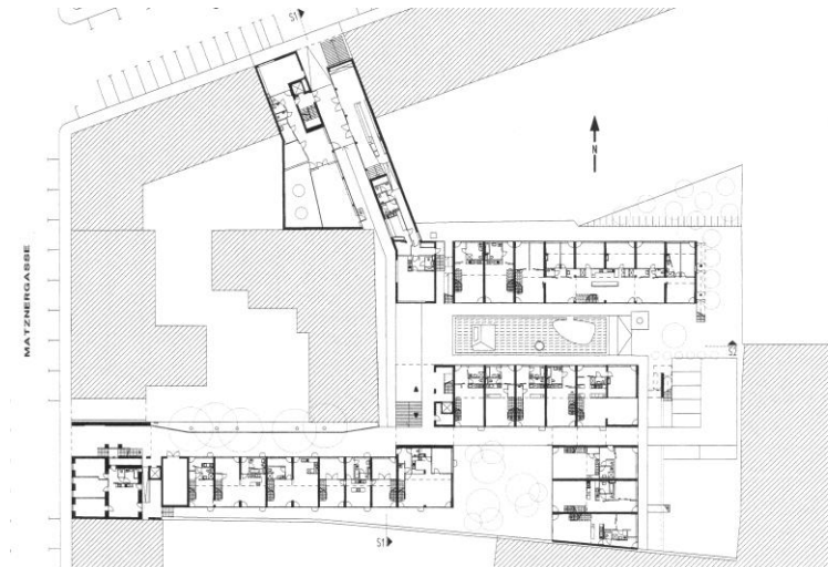
Sargfabrik, Wien 14, bkk 2, 1989-1996, Hof, EG-Grundriss, Kindergruppe, Badehaus
