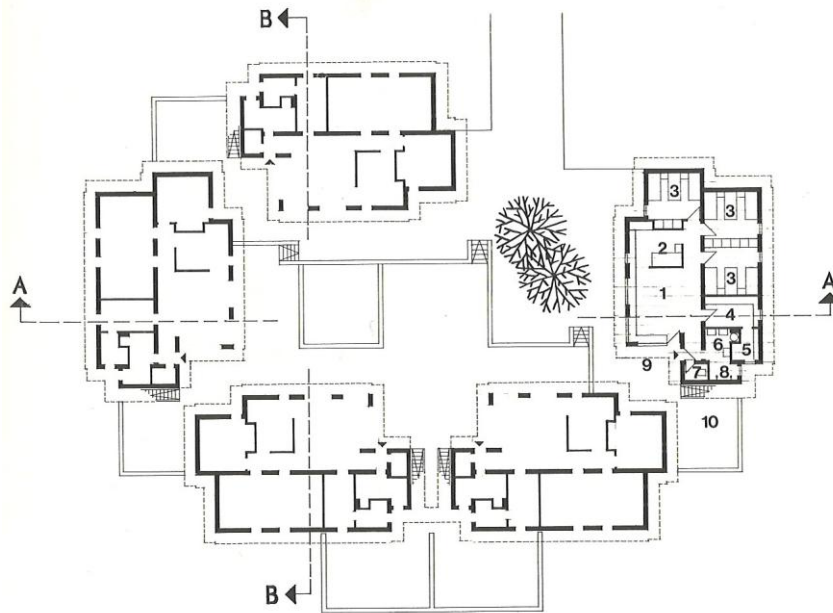
Grundriß Familienhaus 1: 500
