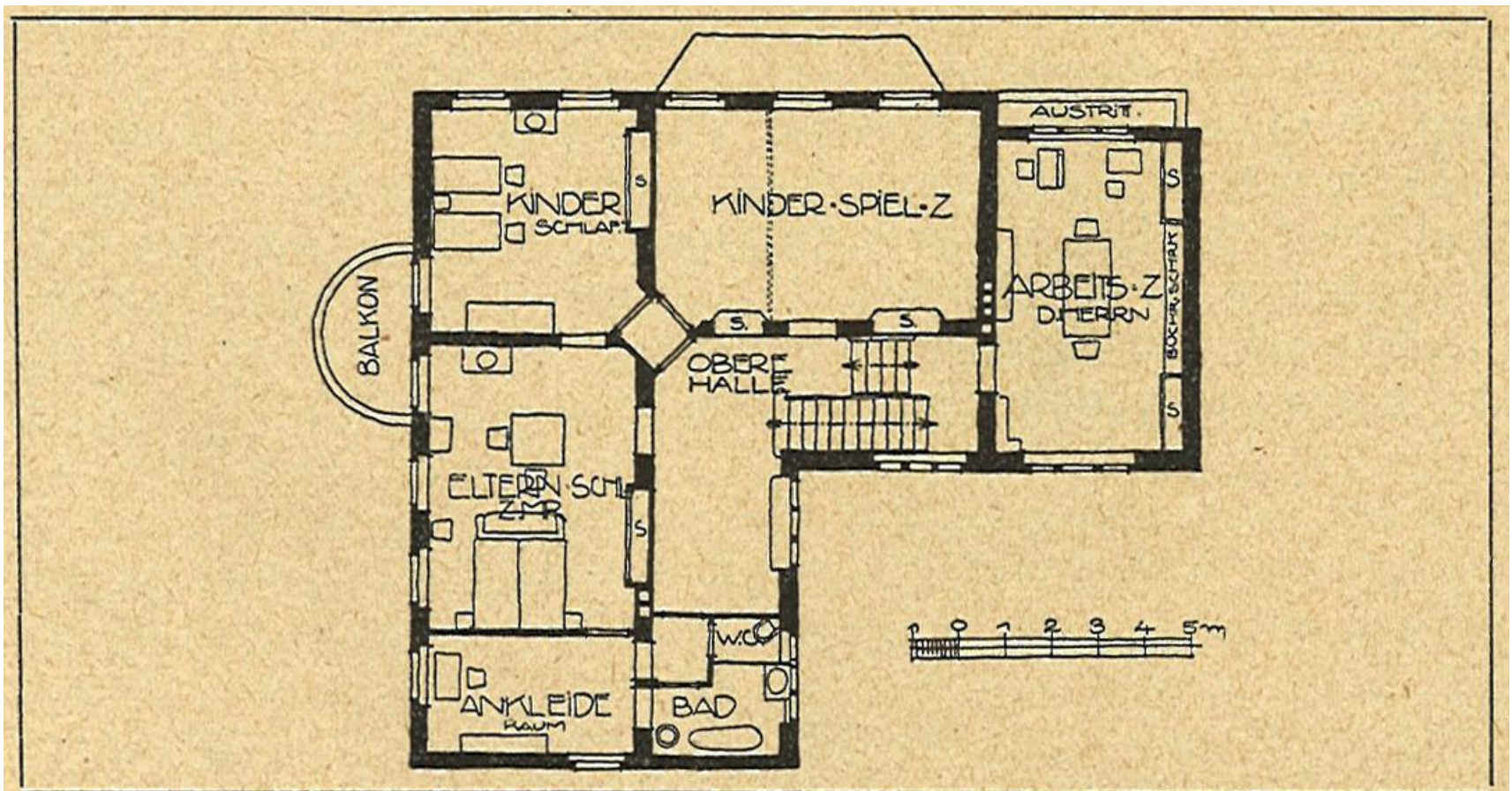
Abb.150. Schlafzimmersgeschoß mit aufteilungsfähigem Kinderzimmer
