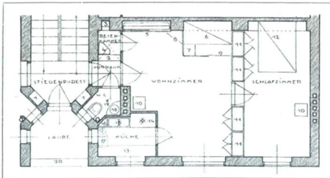
Planverfassung Architekt Anton Brenner. — Ausführung Wiener Stadtbauamt Oben: Volkswohnhaus mit eingebauter Einrichtung Unten: Grundriß des Wohnungstyps im Volkswohnhaus mit eingebauter Einrichtung
