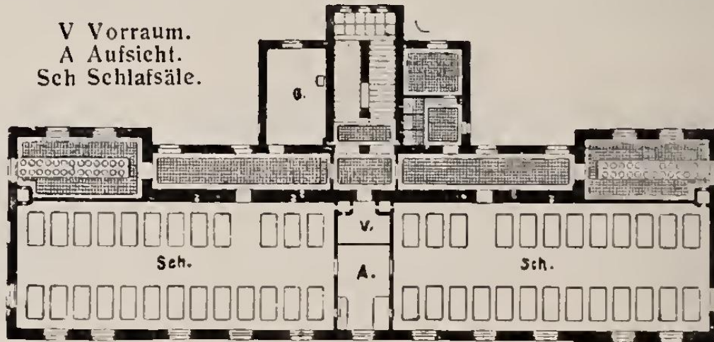
Abb. 386. Waisenhaus für israelitische Mädchen, XIX., Feldgasse. Zweiter Stock. 1 : 600.
