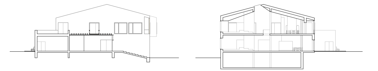
schnitt 1-1 bibliothek _ schnitt 2-2 volksschule _ 1:500
