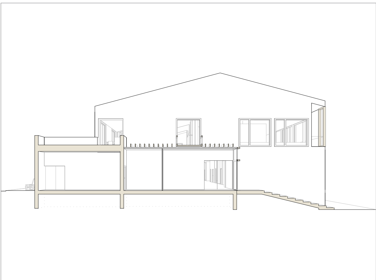
schnitt bibliothek
