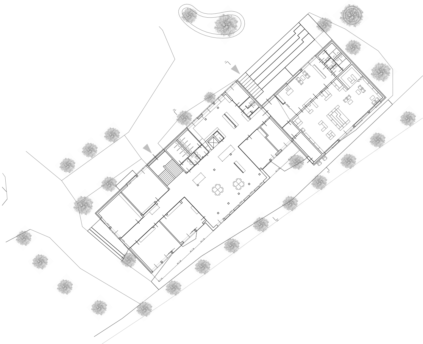
grundriss erdgeschoss volksschule + bibliothek _ 1:500
