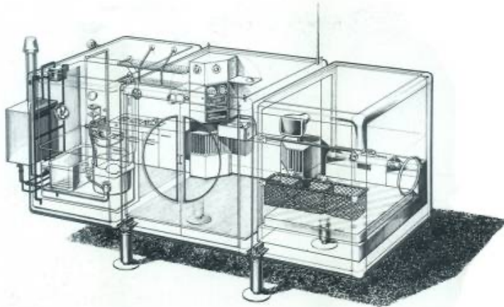
174 Vorfabriziertes Kapselhaus, LC-30X, Japan, Isometrie
